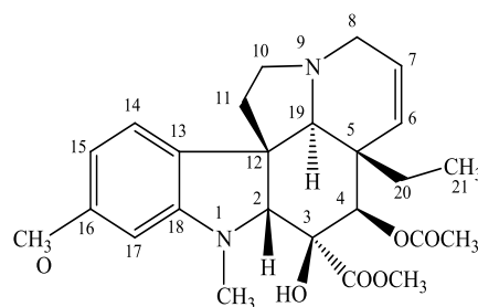
6. vindoline
