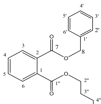
1. spatozoate
