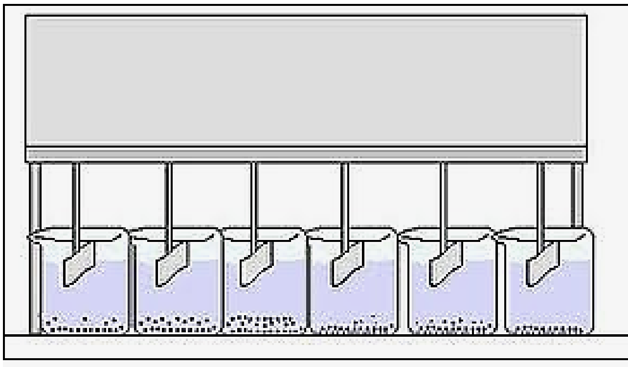
Fig. 2. Jar test Apparatus.
